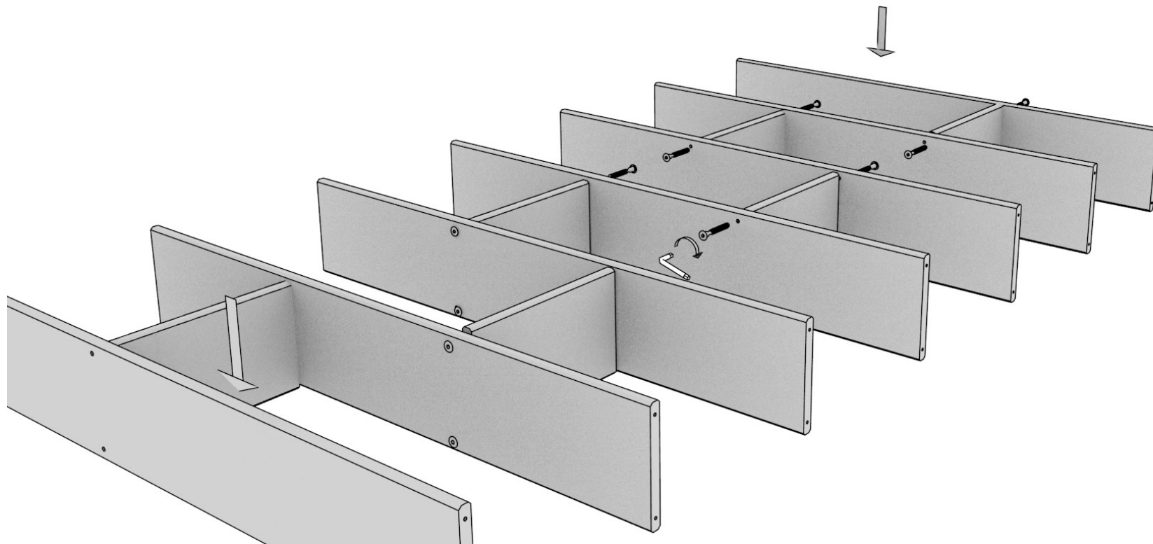
ESTANTERIA ASIMETRICA-7
